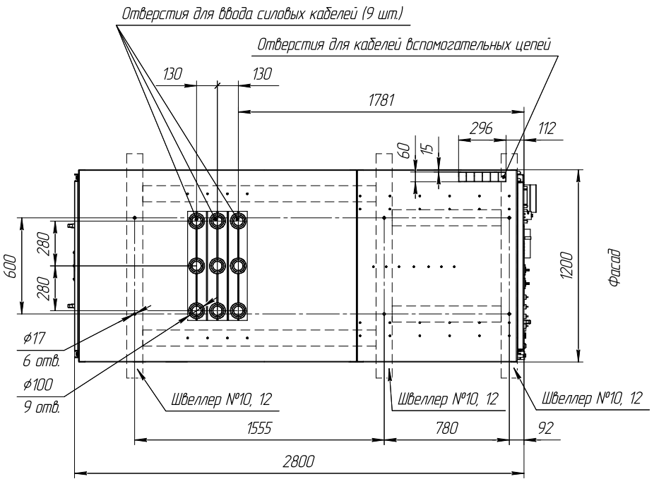
Места крепления ячейки и ввод кабелей К-3.1 2800
